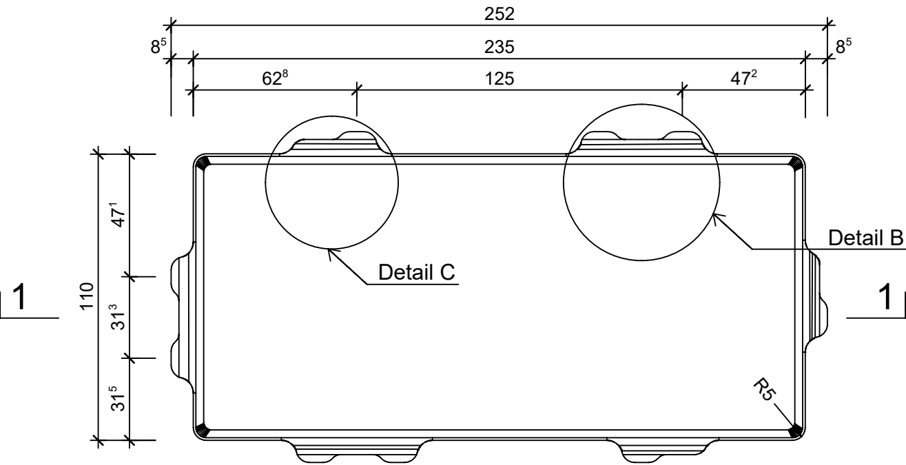
Grundriss, 1:2
