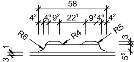
Detail C, 1:2
