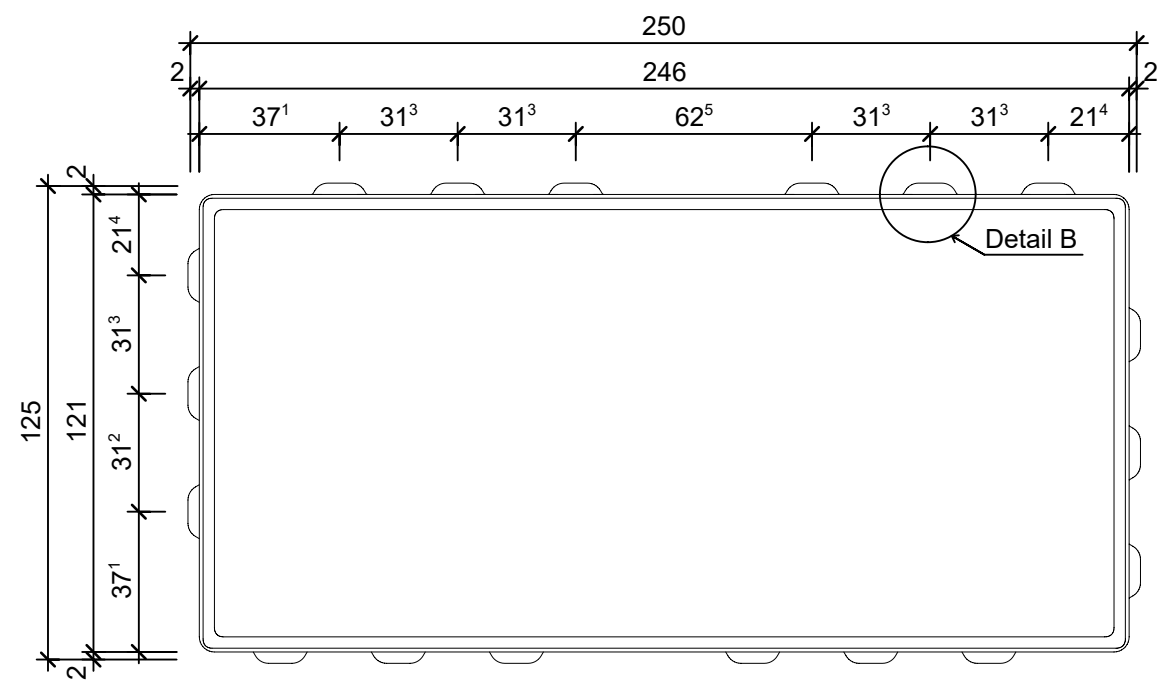
Grundriss, 1:2
