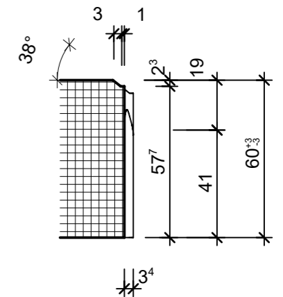
Schnitt 3-3, 1:2
