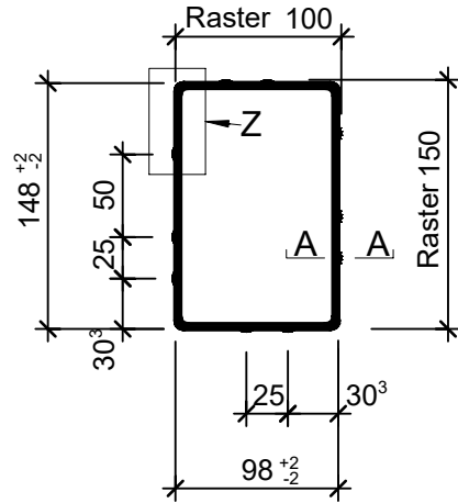
Grundriss, 1:5
