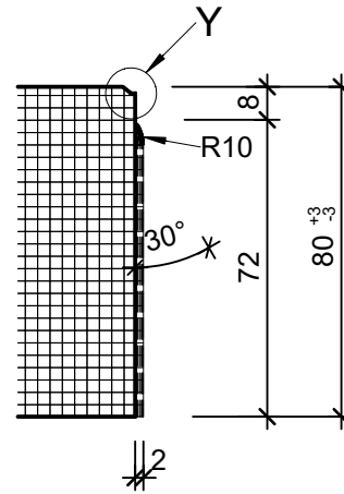
Schnitt A-A, 1:2
