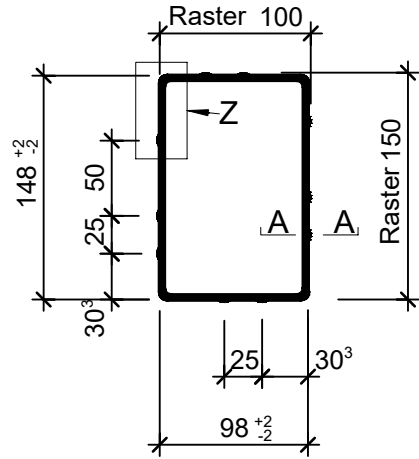
Grundriss, 1:5
