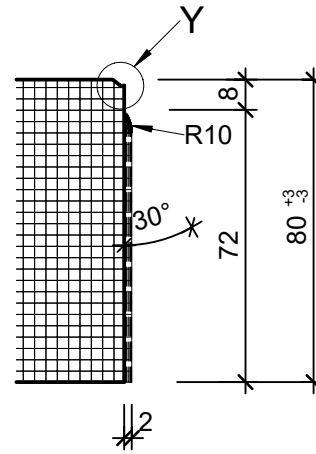
Schnitt A-A, 1:2
