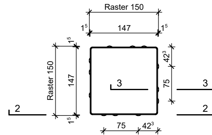
Grundriss 1:5
