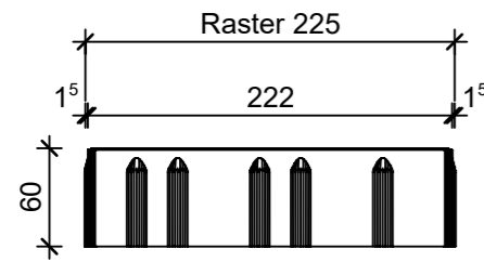
Schnitt 1-1, 1:5
