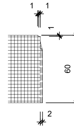
Schnitt 3-3, 1:2
