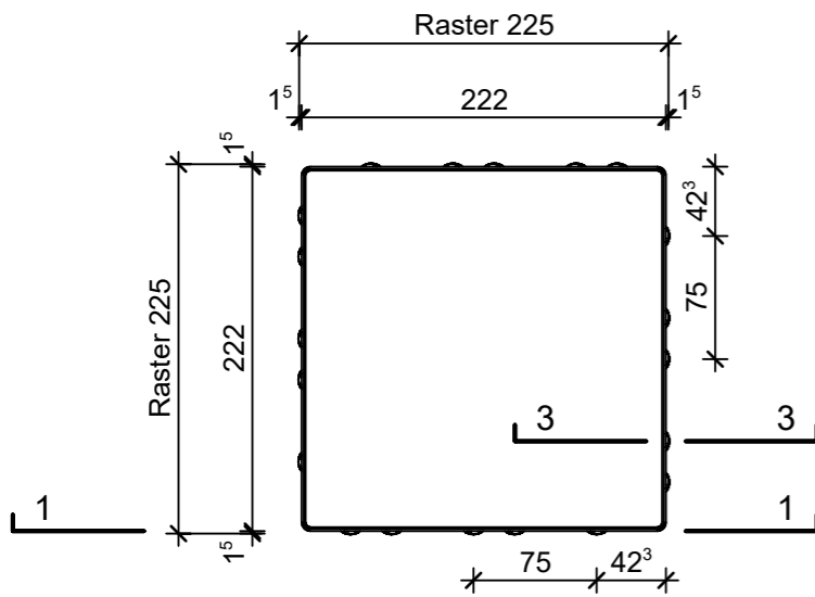
Grundriss 1:5
