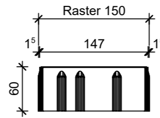
Schnitt 2-2, 1:5
