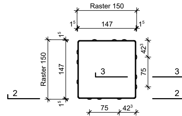
Grundriss 1:5
