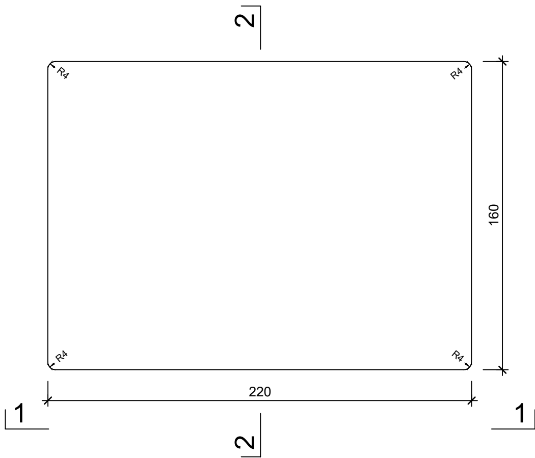
Grundriss, 1:2
