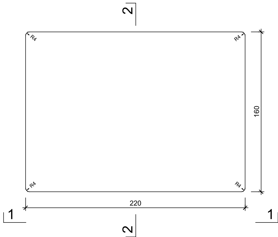
Grundriss, 1:2
