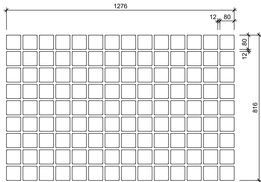
Grundriss, 1:2
