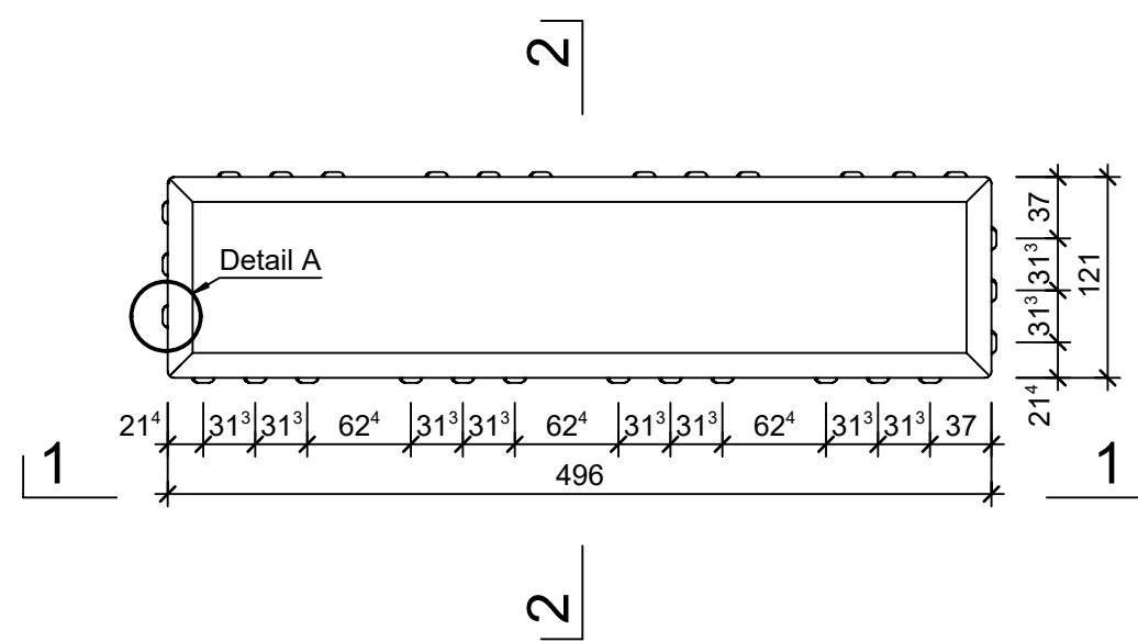
Grundriss, 1:5
