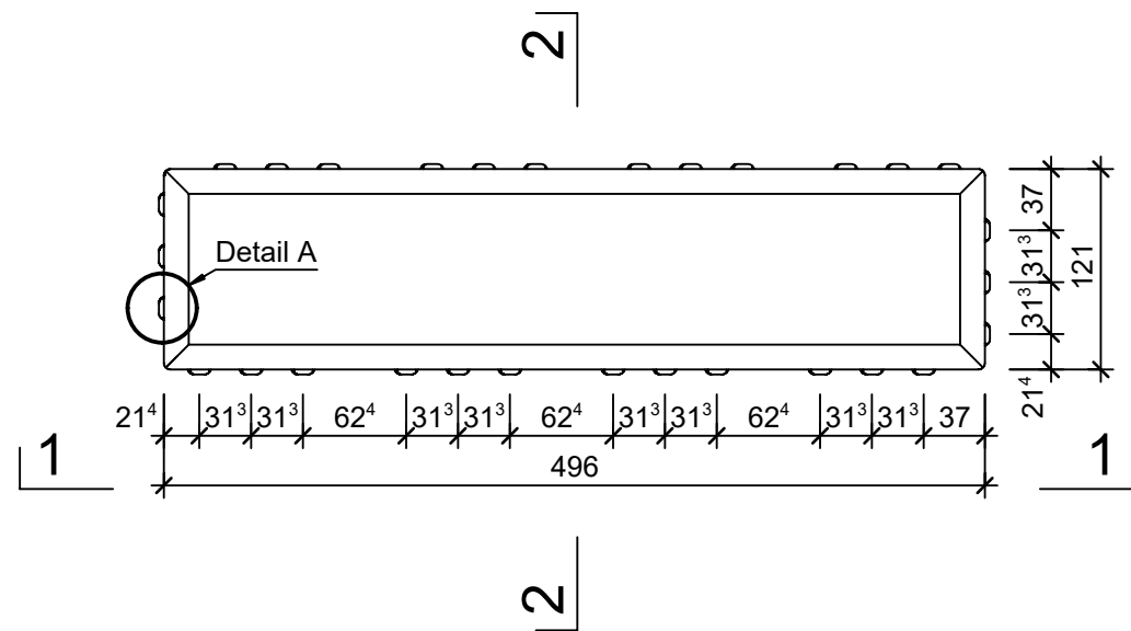
Grundriss, 1:5
