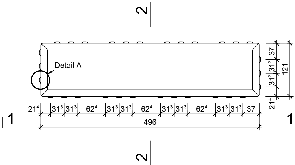
Grundriss, 1:5
