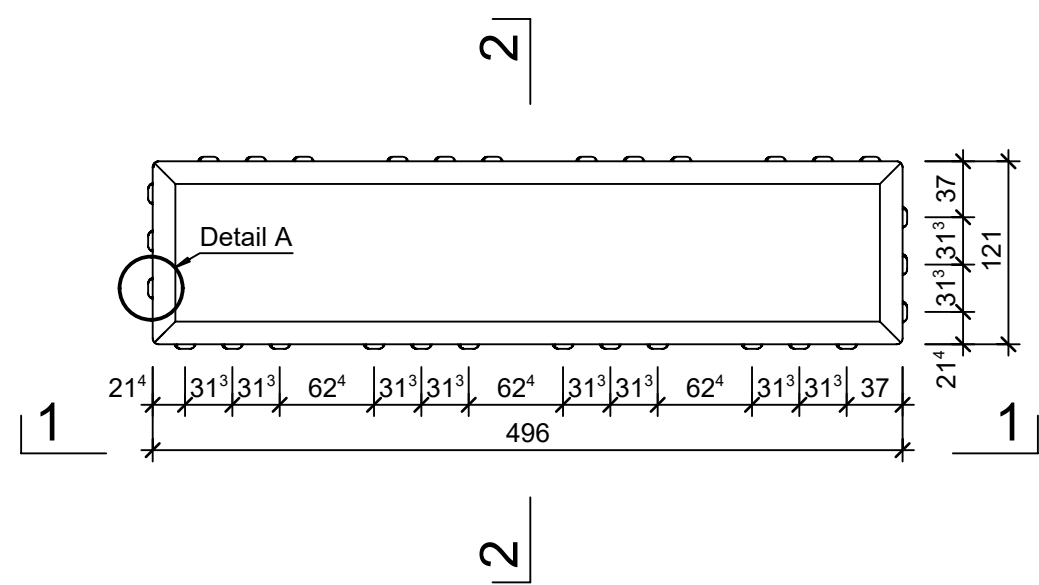
Grundriss, 1:5
