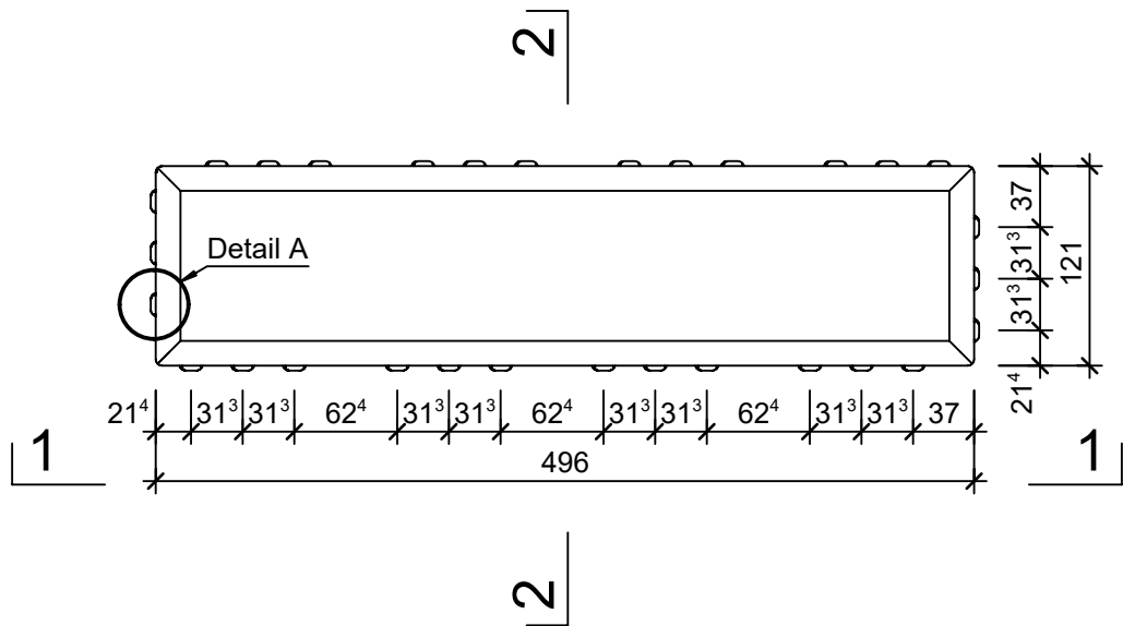
Grundriss, 1:5
