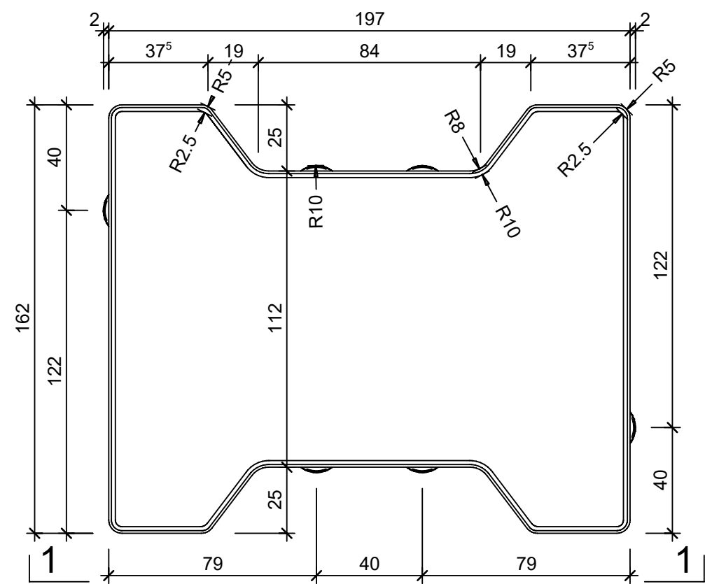
Grundriss, 1:2
