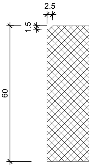
Schnitt 2-2, 1:1
