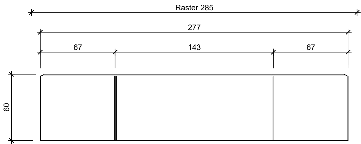
Schnitt 1-1, 1:2
