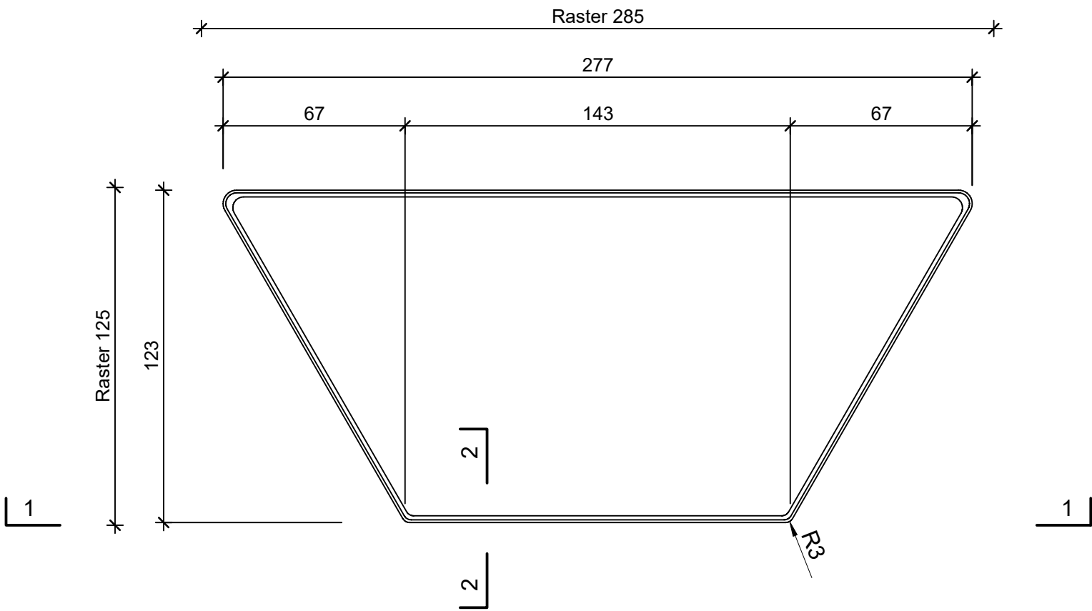
Grundriss 1:2
