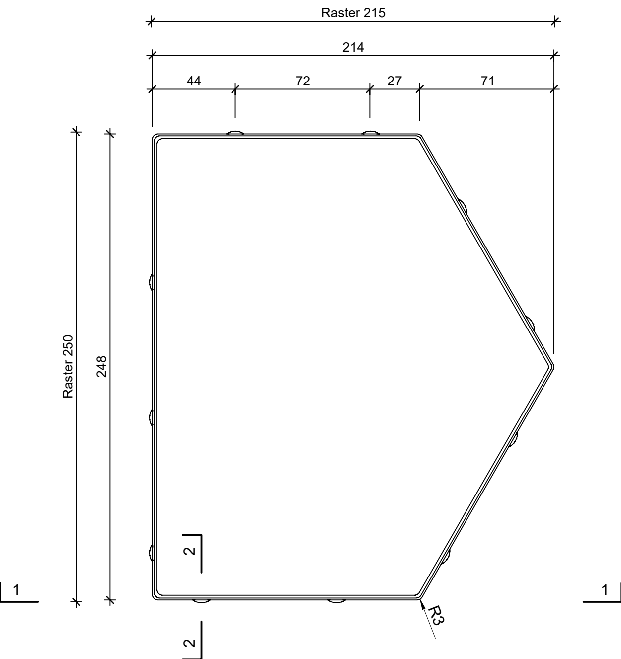
Grundriss 1:2
