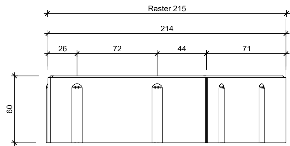
Schnitt 1-1, 1:2
