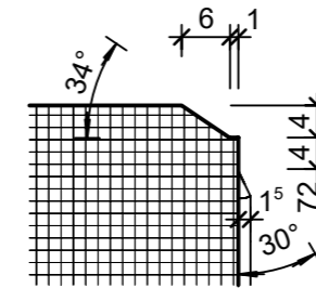
Schnitt 2-2, 1:1
