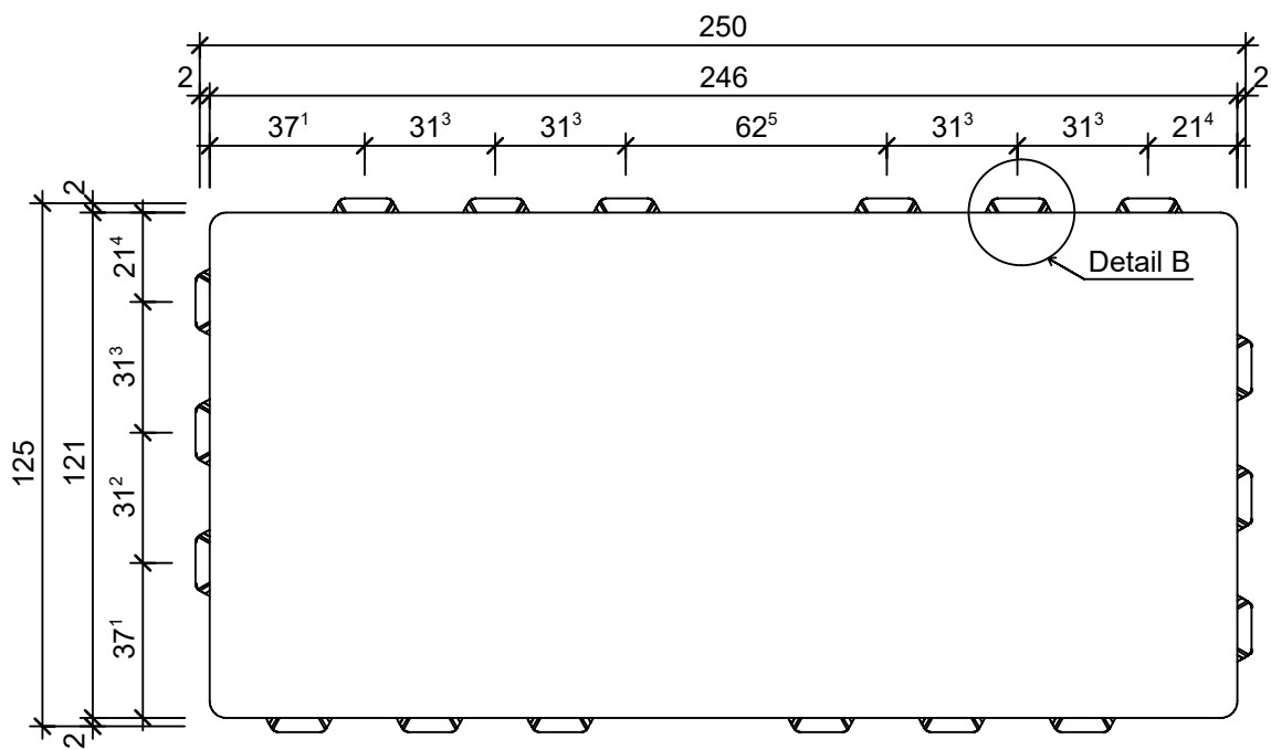
Grundriss, 1:2
