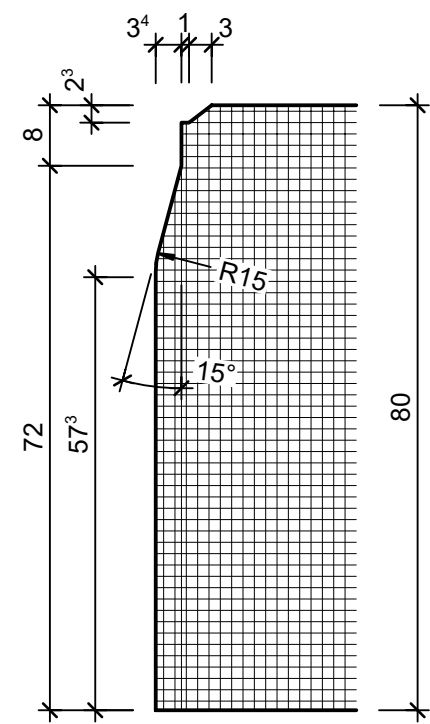
Detail A, 1:1
