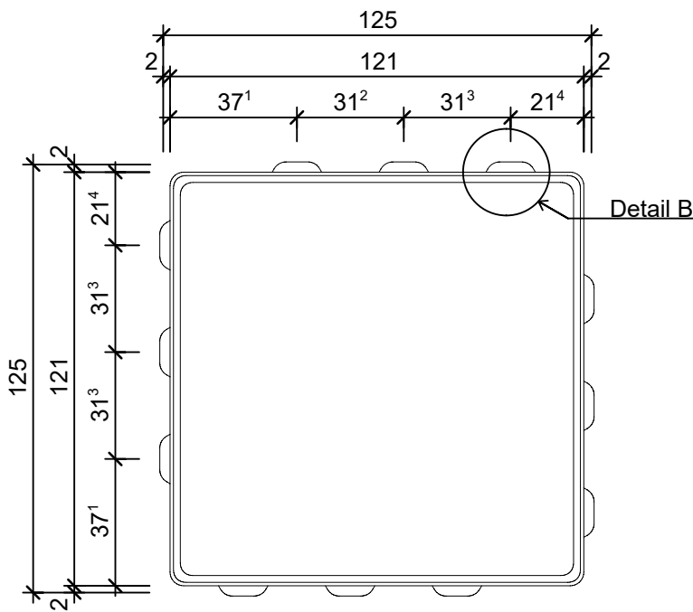
Grundriss, 1:2
