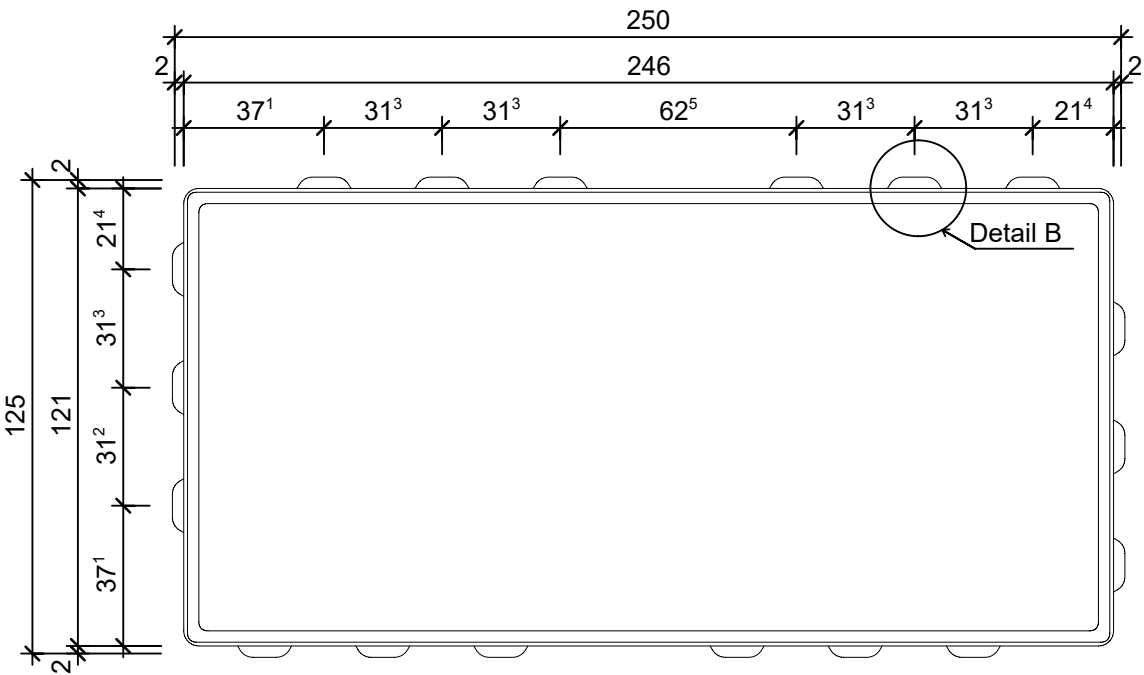
Grundriss, 1:2
