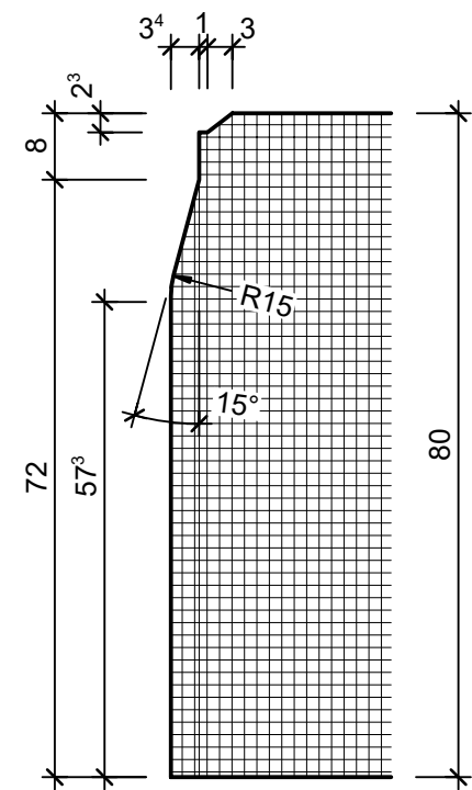
Detail A, 1:1
