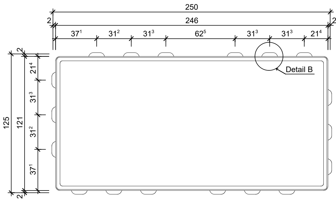
Grundriss, 1:2
