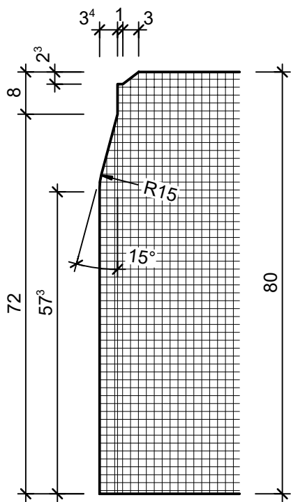
Detail A, 1:1
