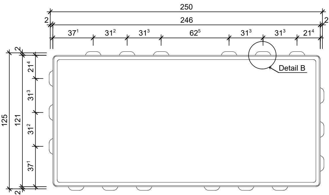
Grundriss, 1:2
