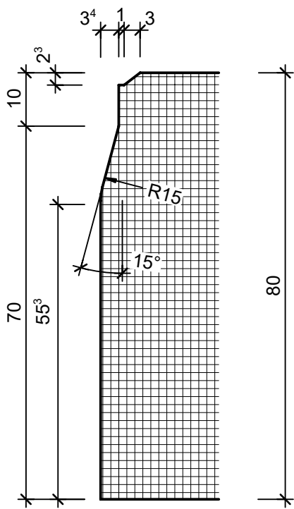
Detail A, 1:1
