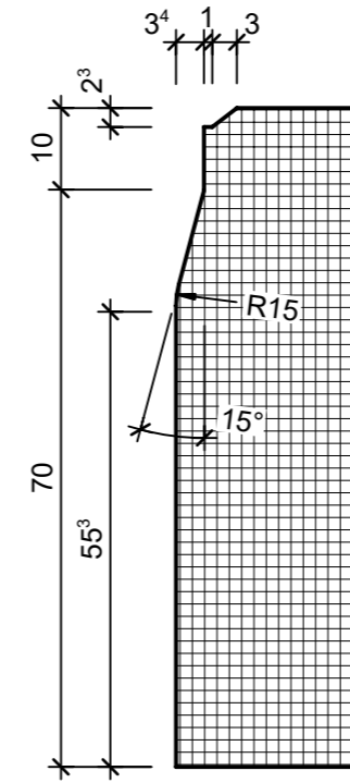
Detail A, 1:1
