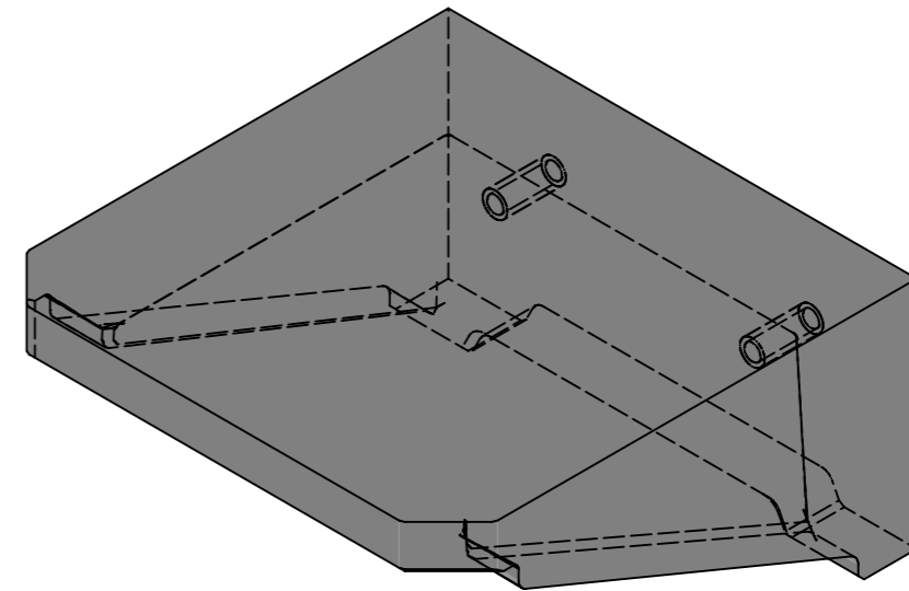
Isometrie, 1:5
