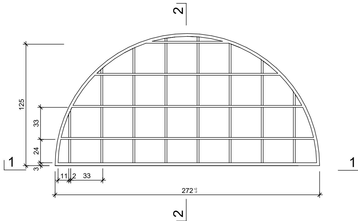
Grundriss, 1:2
