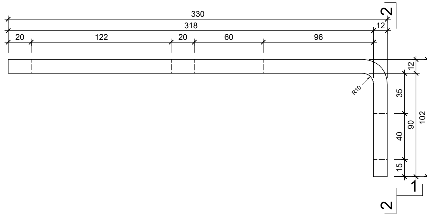
Grundriss 1:2
