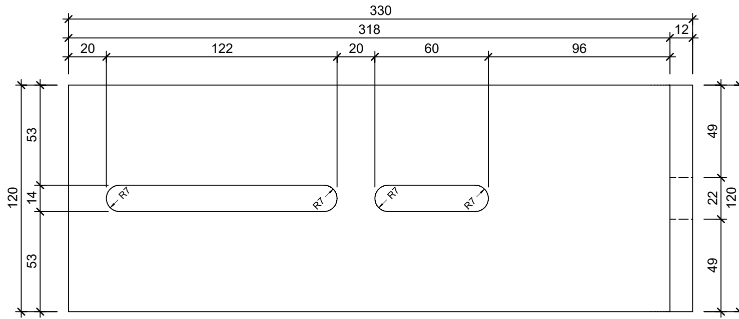
Ansicht 1, 1:2
