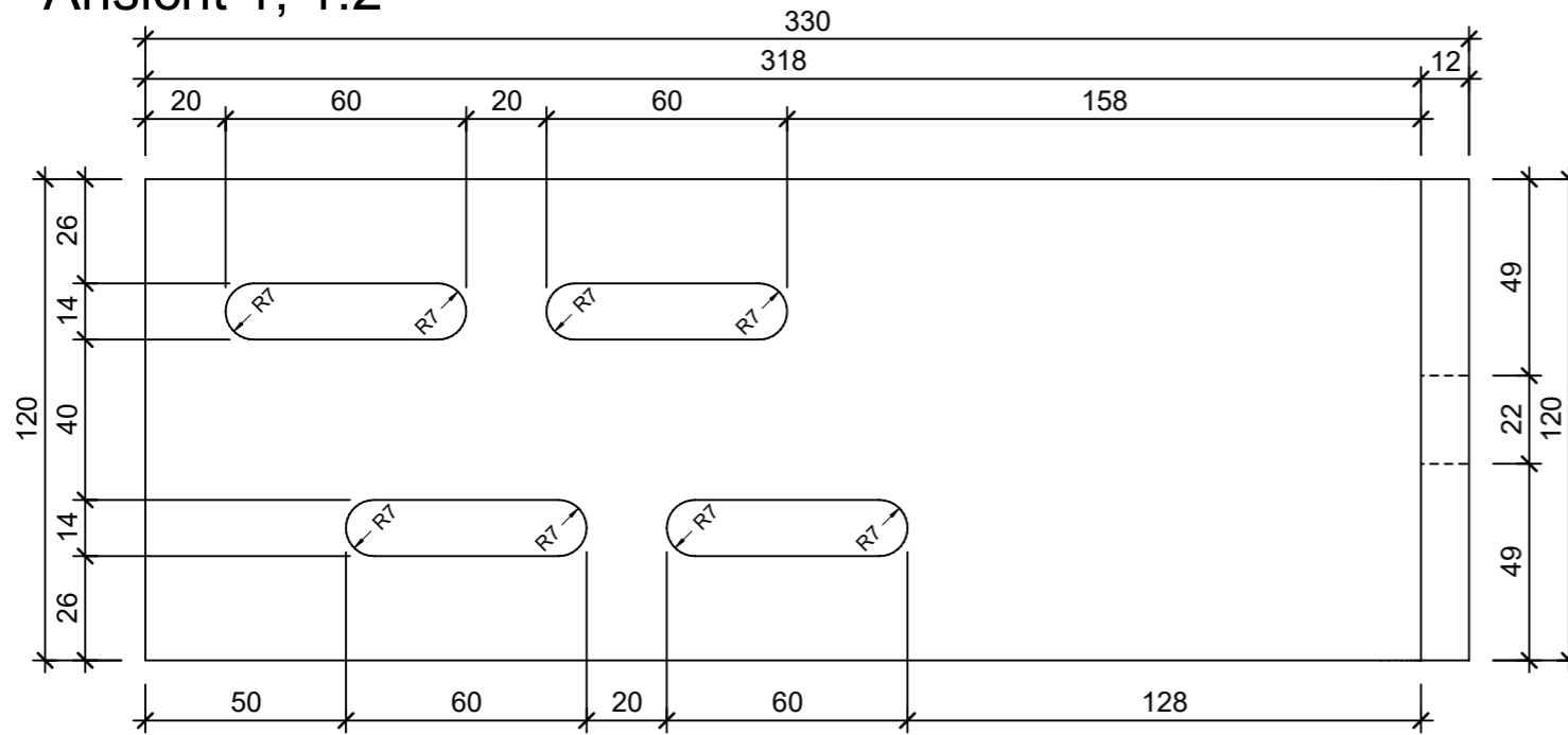
Ansicht 1, 1:2
