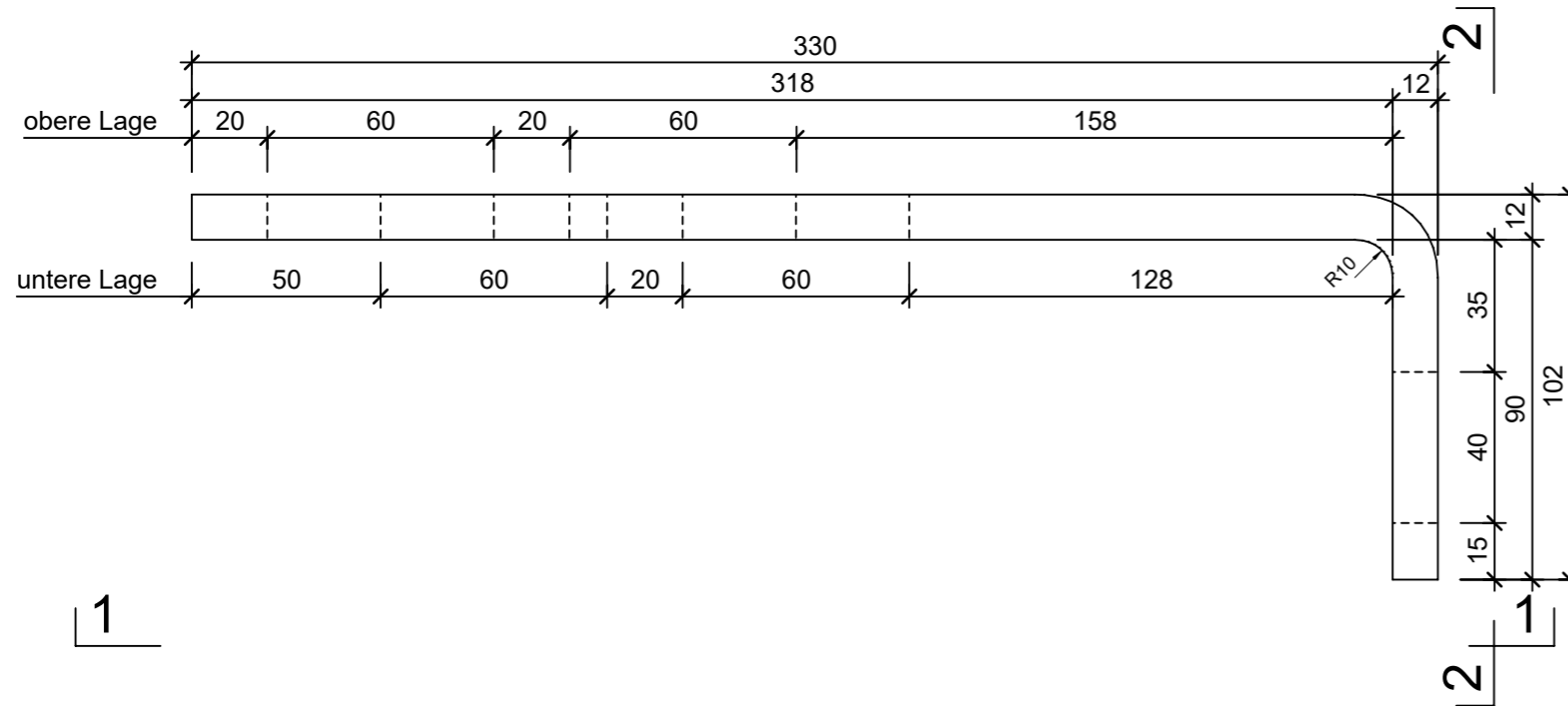
Grundriss 1:2
