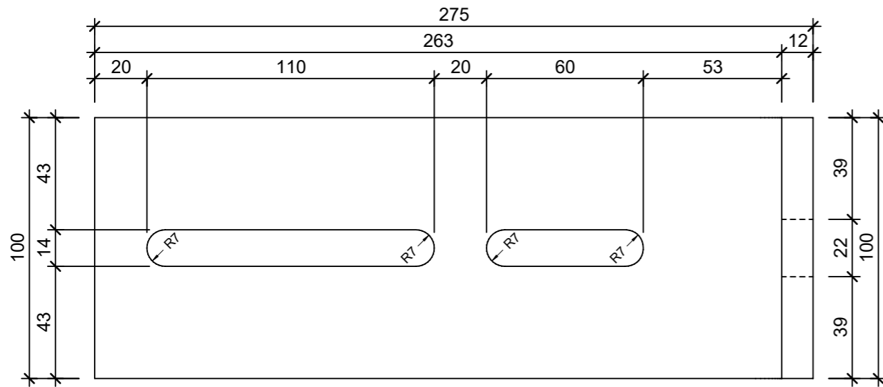
Ansicht 1, 1:2
