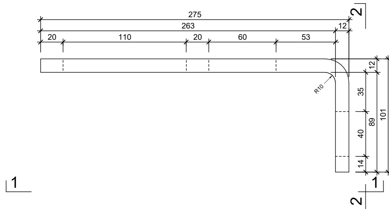
Grundriss 1:2
