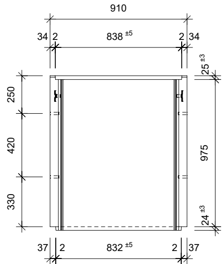
Ansicht 1-1, 1:25
