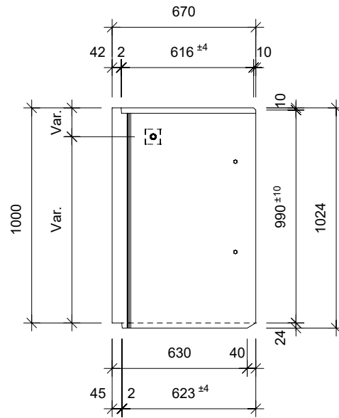
Schnitt 2-2, 1:25
