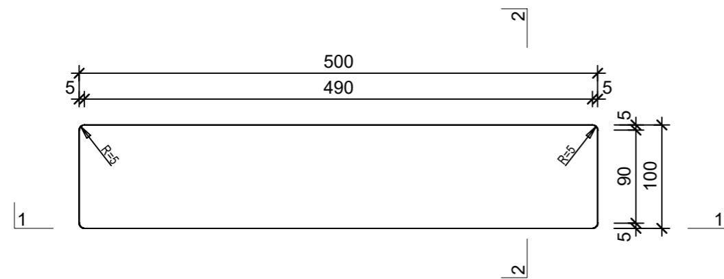
Grundriss, 1:5
