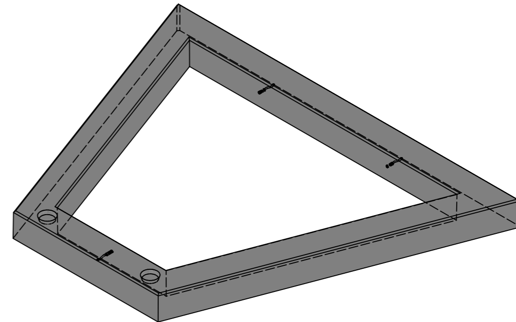
Isometrie, 1:20
