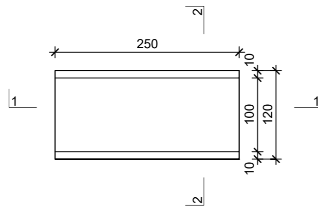
Grundriss, 1:5
