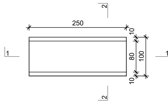
Grundriss, 1:5
