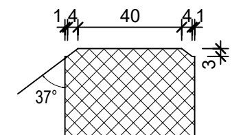
Detail A, 1:2
