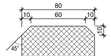
Detail A, 1:2
