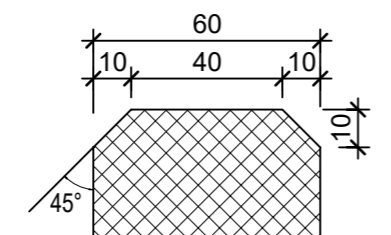
Detail A, 1:2
