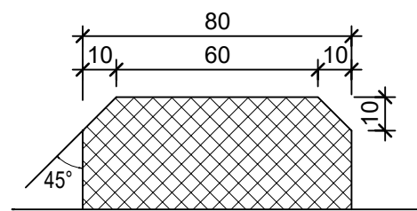
Detail A, 1:2
