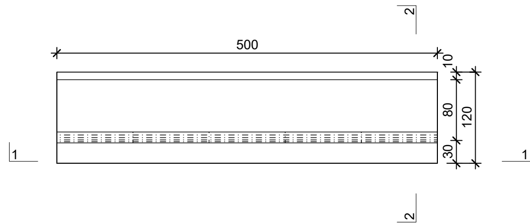
Grundriss, 1:5
