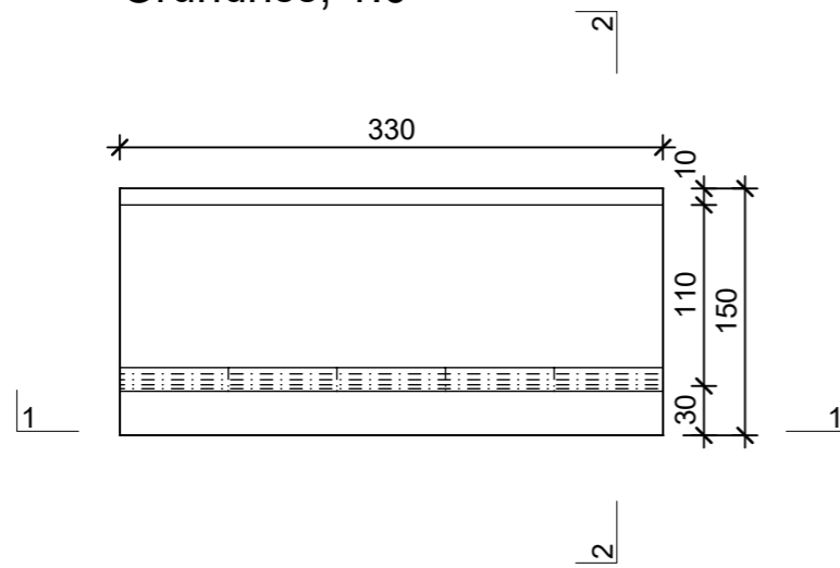
Grundriss, 1:5
