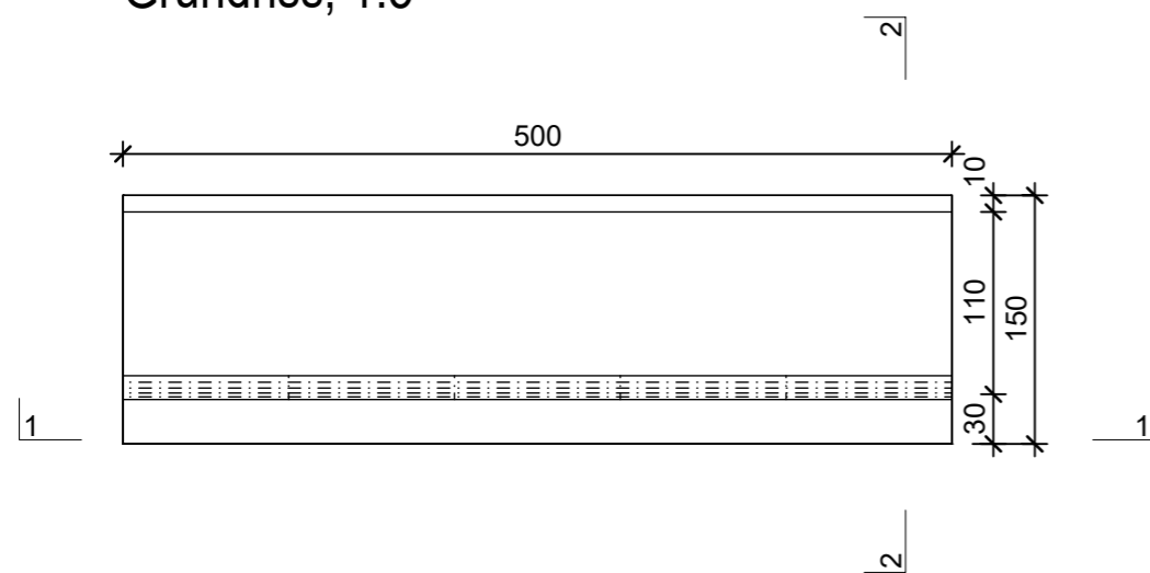
Grundriss, 1:5
