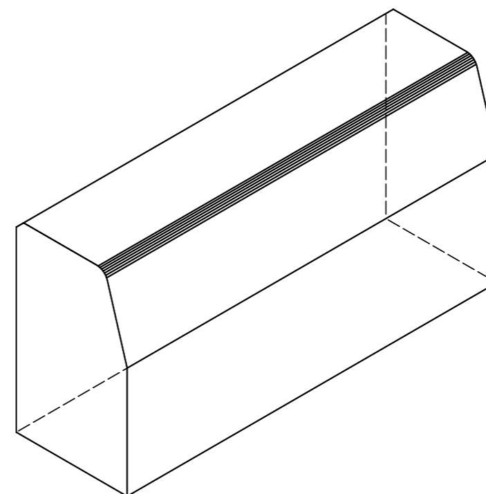
Isometrie, 1:5
