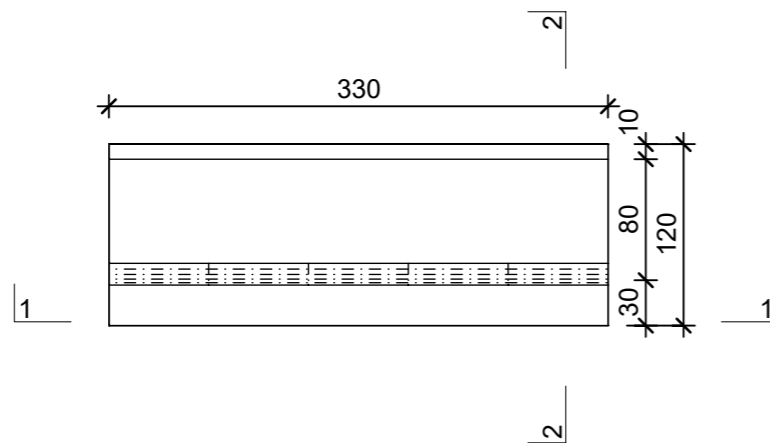
Grundriss, 1:5
