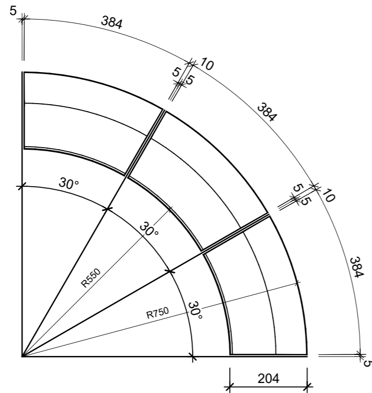
Grundriss, 1:5
