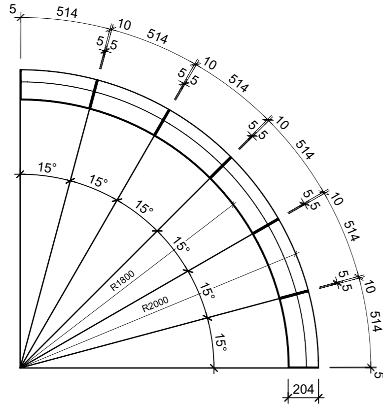
Grundriss, 1:5
