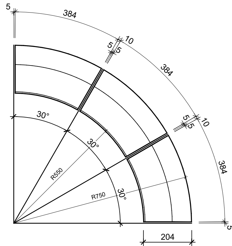
Grundriss, 1:5
