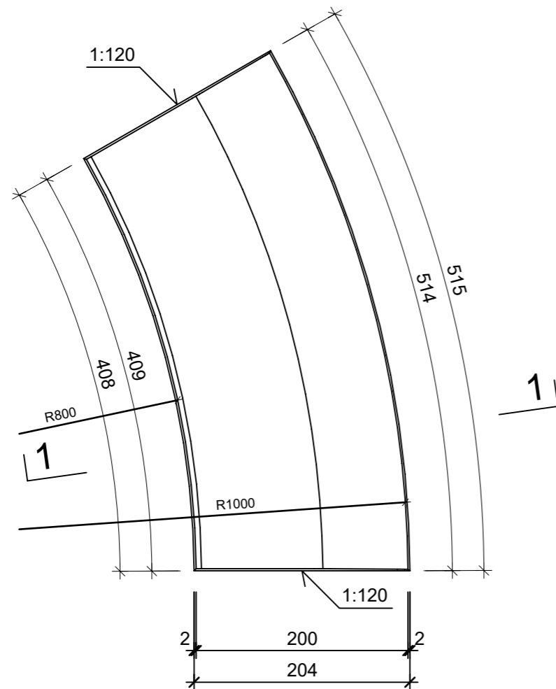
Grundriss, 1:5
