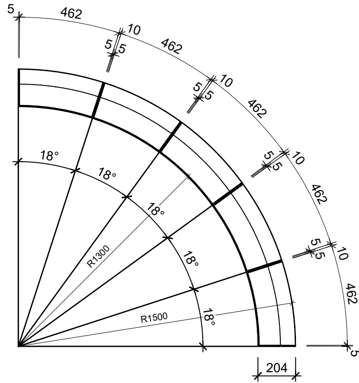
Grundriss, 1:5
